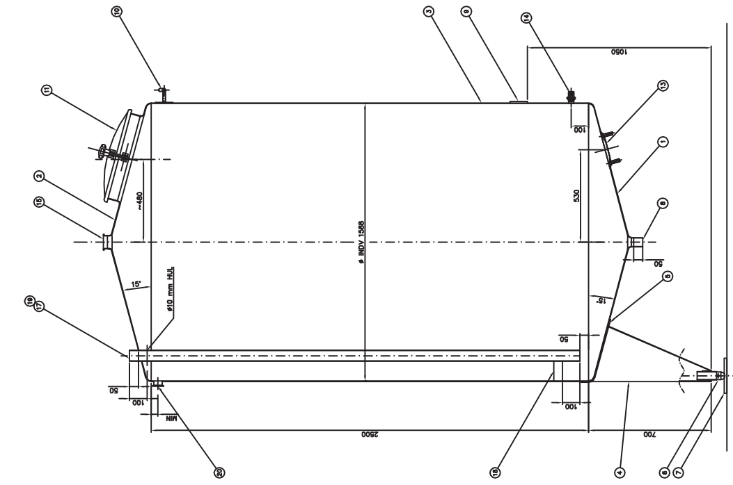
LODRET SNIT
